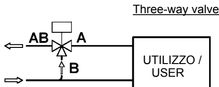
Fig. 2 Miscelazione a portata variabile all'utilizzo / Variable flow mixing to the user.
